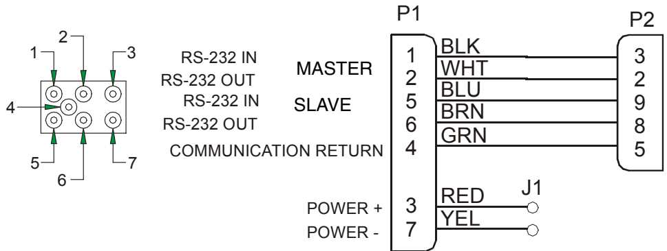
RDI ADCP WH I/O Cable
