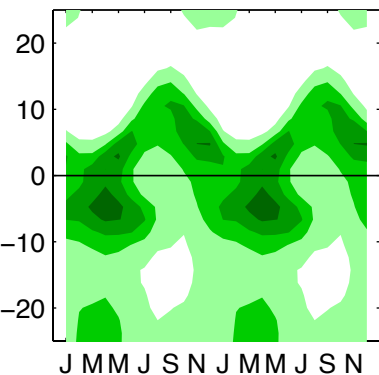
CCM3
