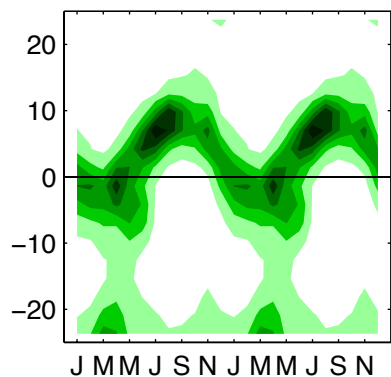
GFDL_R30
