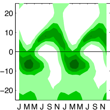
NSIPP
