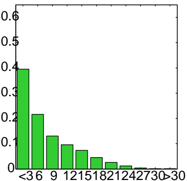
CCM3
