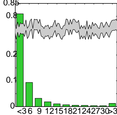
GFDL_R30
