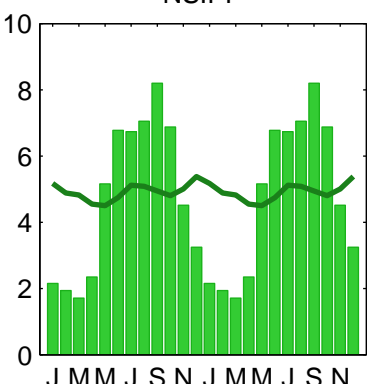
NSIPP
