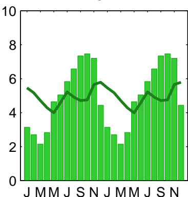
CCM3
