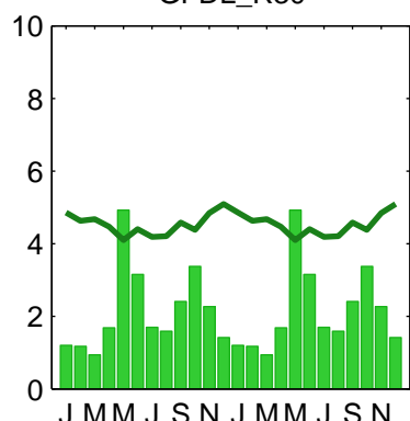
GFDL_R30
