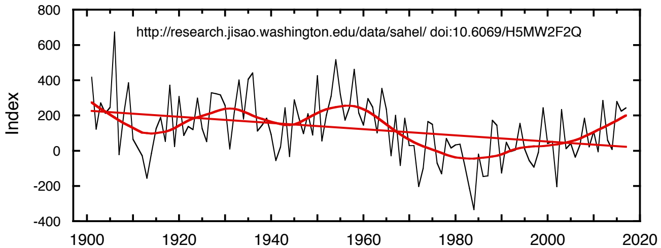
HadISST SSTs
