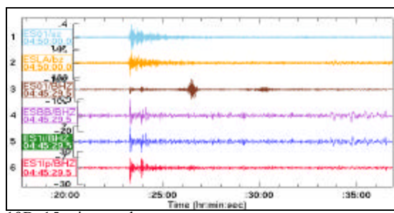
19B. 15 min raw data
