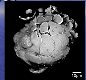
SEM photo of FeNiCr
