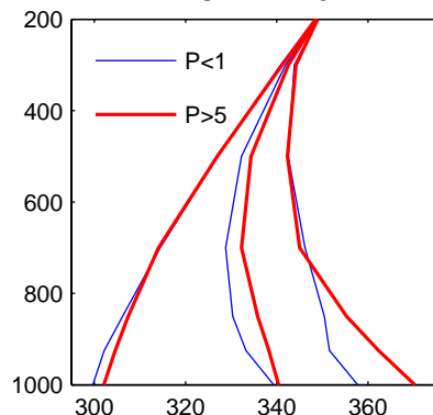
ECHAM 4.5
