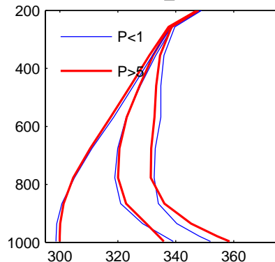
GFDL_R30
