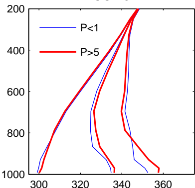
CCM3
