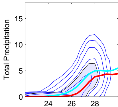
CCM3
