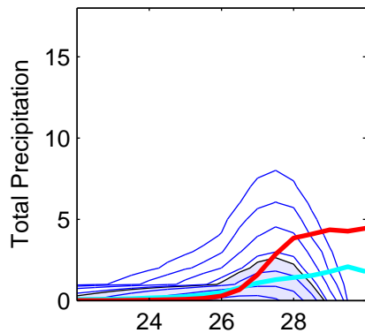
GFDL_R30
