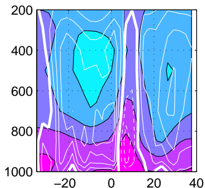
GFDL_R30
