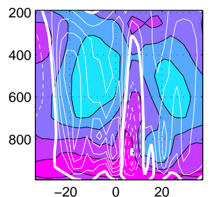
NSIPP
