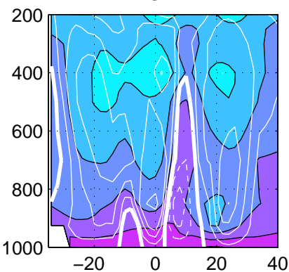
NSIPP
