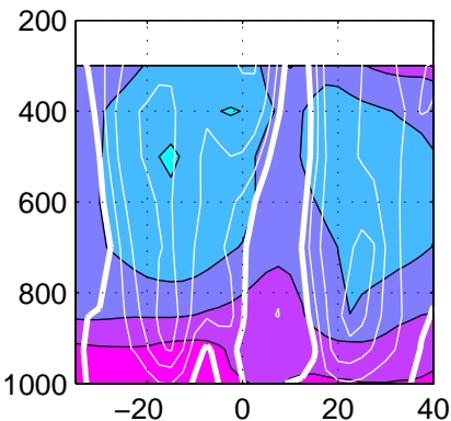
CCM3
